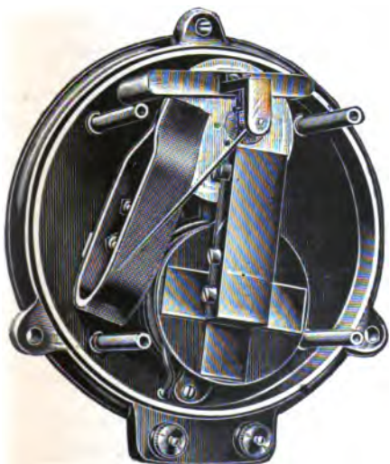
Abb. 439. Induktionsinstrument (Strom- oder Spannungsmesser) der Allgem. Elektrizitäts-Gesellschaft.
